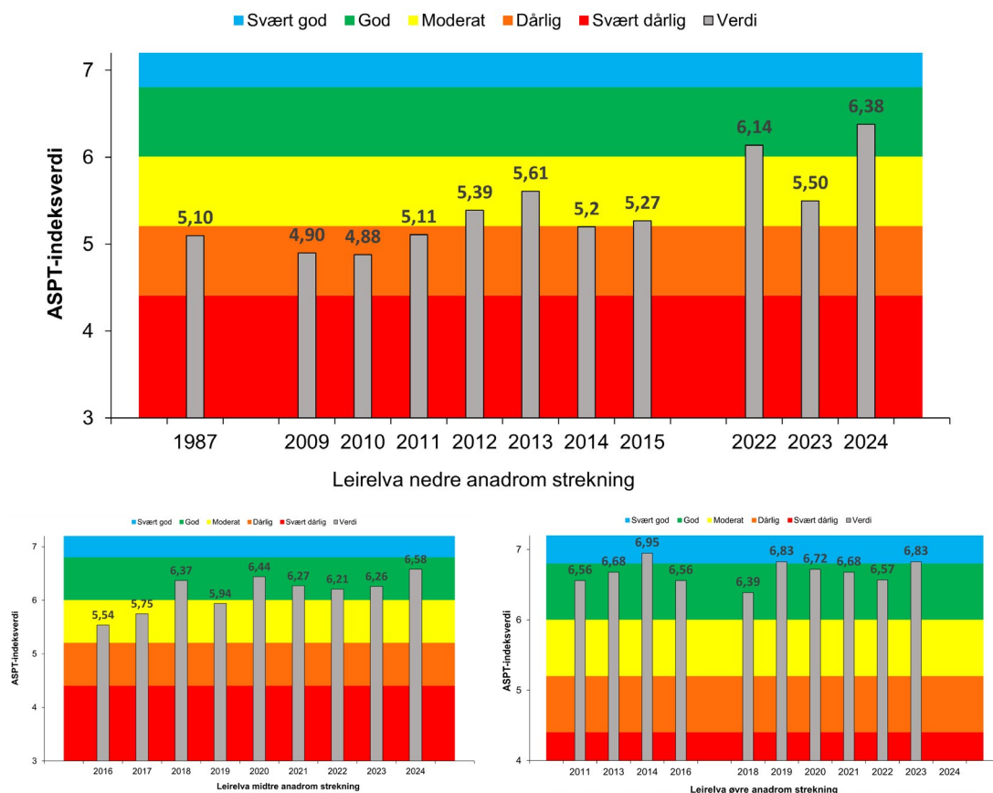
Figur 5. ASPT-verdier fra bunndyrprøver i øvre, midtre og nedre del av anadrom strekning i Leirelva i perioden 1987-2024. Bakgrunnsfarger etter femdel skala for økologisk tilstand. Grensenivå for miljømål og «God økologisk tilstand» er 6,0.
