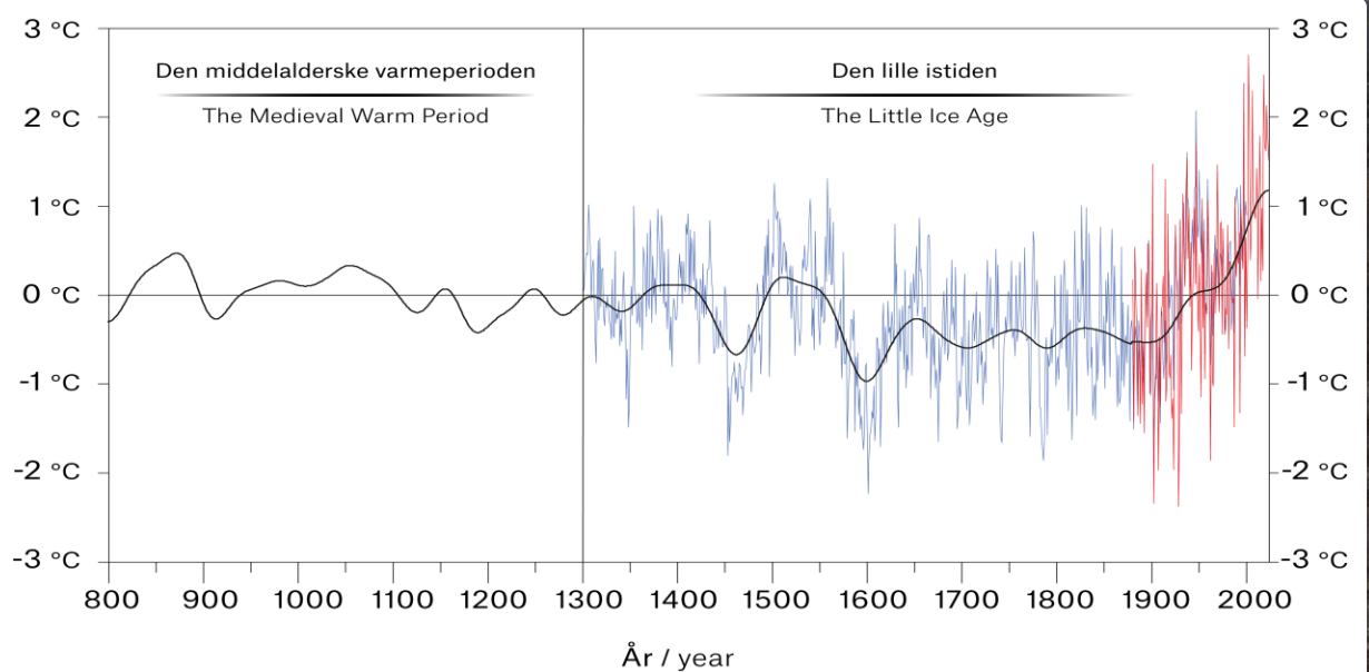
Rekonstruerte sommertemperaturer i Skandinavia angitt som avvik fra den moderne referanserammen (1961-1990). Graf utviklet av Fredrik C. Ljungqvist.
