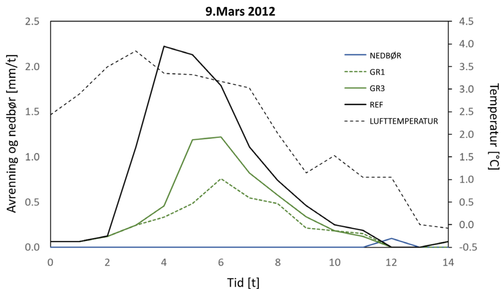
Figur 2. Snøsmelting og avrenning fra det tradisjonelle taket (REF) og de to grønne takene (GR) fulgte lufttemperaturene ganske tett. Snødybden gikk ned fra 5 cm i begynnelsen av episoden til 0 cm på slutten. Den relative reduksjonen i avrenning var 66 % for GR1 og 45 % for GR3. Gjennomsnittlig vanninnhold i substratet var 20 og 25 % for henholdsvis GR1 og 3. Feltkapasiteten til de grønne takene ble nådd siden avrenningen hadde startet før avrenningstoppene.
