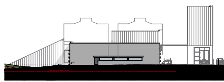
1:200 Fasett nord-øst (plan 0000000000)
