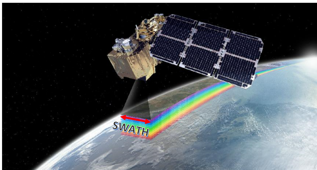
Figur 1. Animasjon av Sentinel-2B satellitten i bane. Lastet ned fra ESAs nettside https://directory.eoportal.org/web/eoportal/satellite-missions/c-missions/copernicus-sentinel-2 . Tekst og rød pil er lagt til for å vise «swath».
